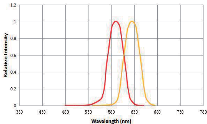
光谱分布特性曲线 Spectrum Distribution ( T_a=25^{\circ}\text{C} )
