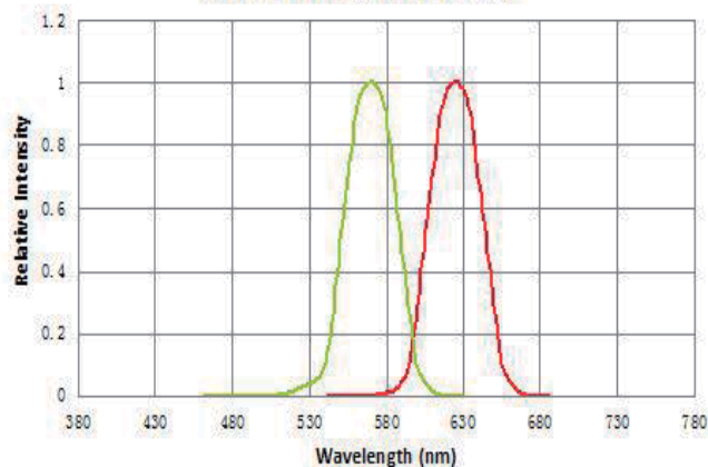
光谱分布特性曲线 Spectrum Distribution ( T_a=25^{\circ}\text{C} )
