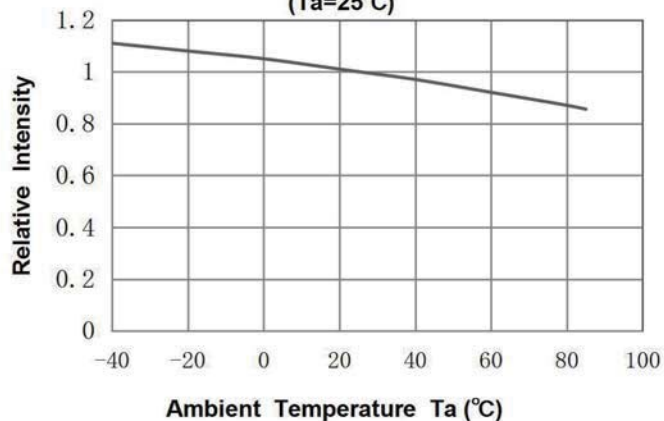
相对光强与环境温度特性曲线 Relative Intensity VS. Ambient Temperature ( T_a=25^{\circ}\text{C} )
