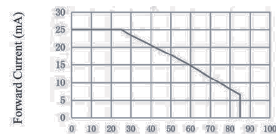
最大正向电流与环境温度特性曲线
