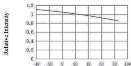
相对光强与环境温度特性曲线
