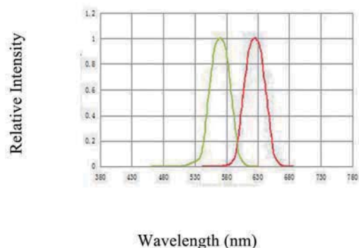
光谱分布特性曲线 Spectrum Distribution (Ta=25°C)
